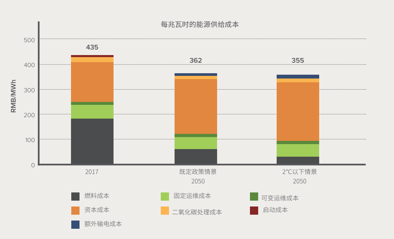
图 34 中国2017和2050年不同情境下的系统成本对比
