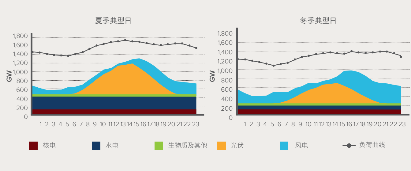
图 25 2030年中国典型冬季和夏季全国电力供需平衡模拟结果 xii
