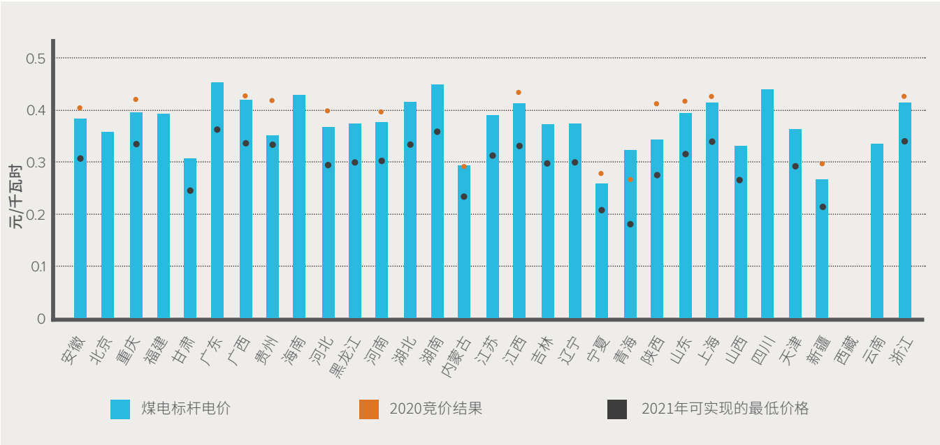
图 8 中国新建煤电、2021年可行价格与2020竞价对比 vii
