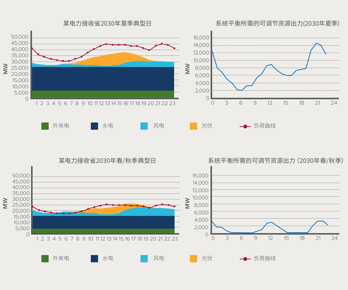
图 27 2030年中国中部地区某电力接收省典型日平衡模拟 xiii
