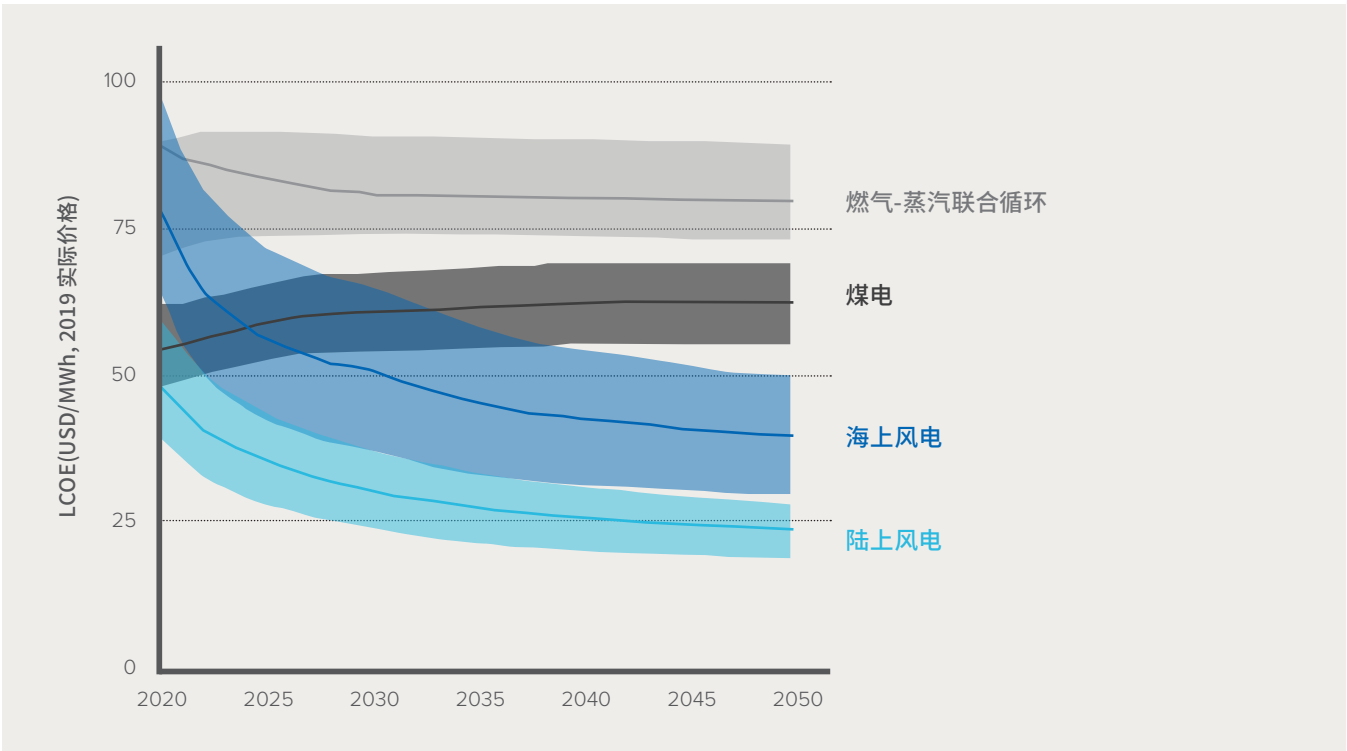
图 11 中国各发电来源新建大规模发电项目经济性对比 15
