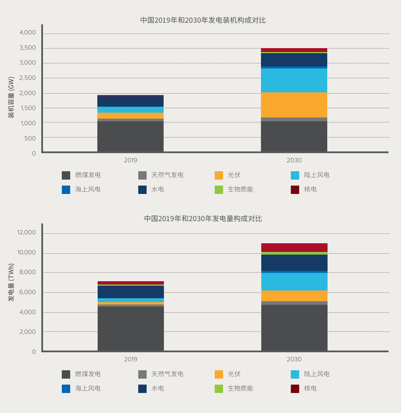
图 2 在零碳投资情景下，中国2030年的发电量和发电装机构成 iii
