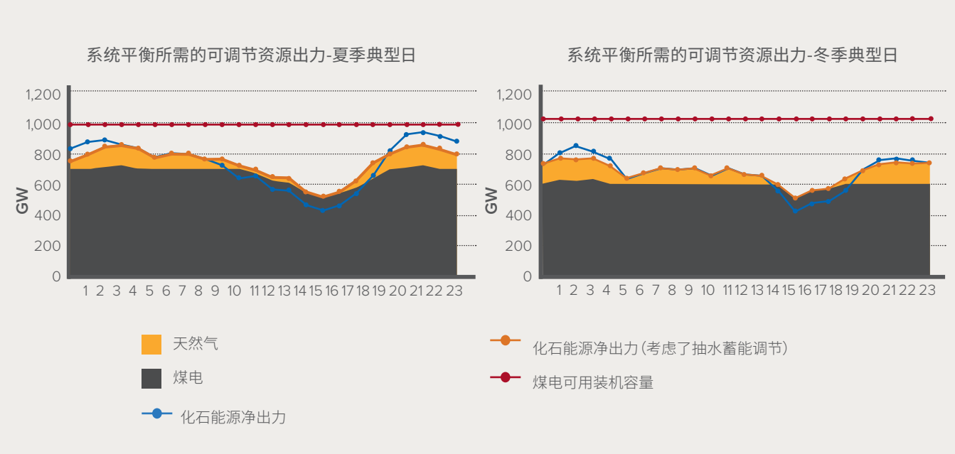
图 26 中国2030电力系统灵活性发电需求
