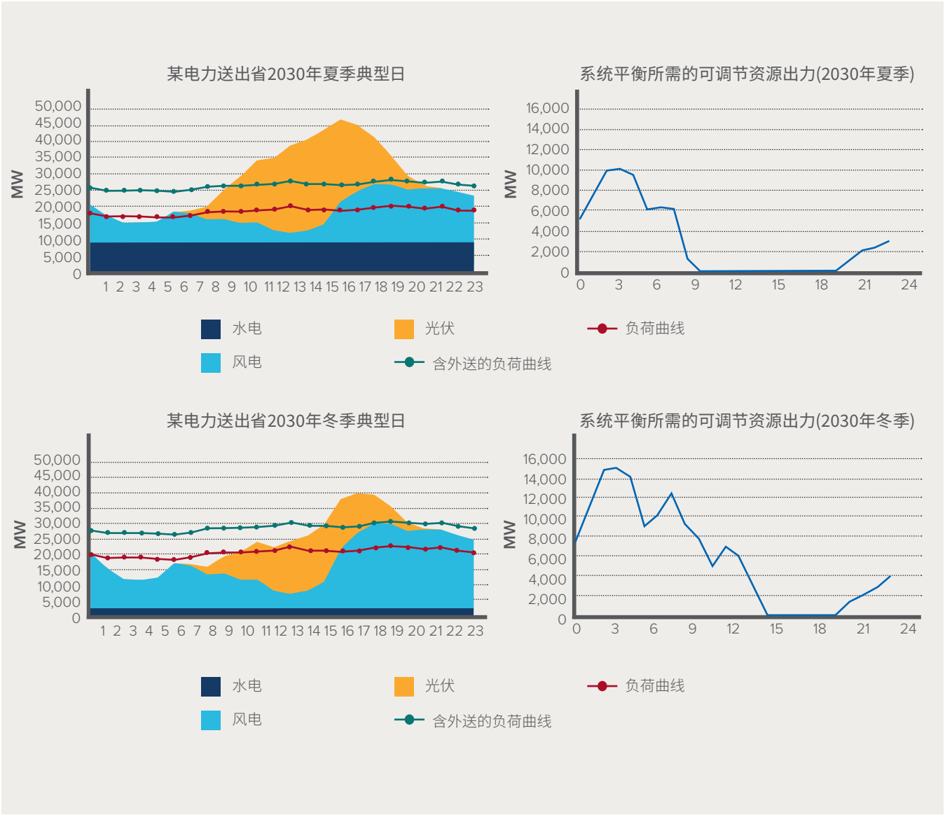
图 28 2030年中国西北部地区某电力输出省典型日平衡模拟
