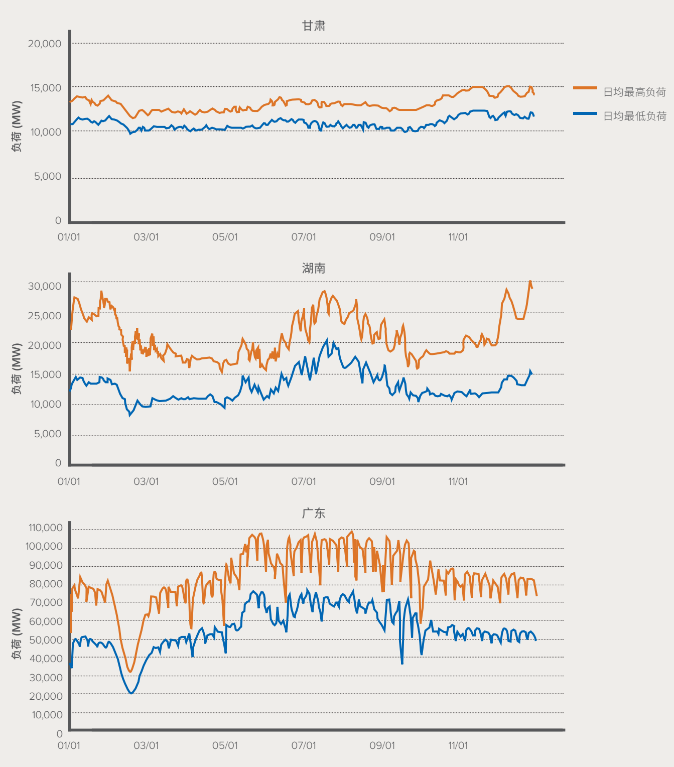
图 22 2019年中国三个省份的典型年负荷曲线
