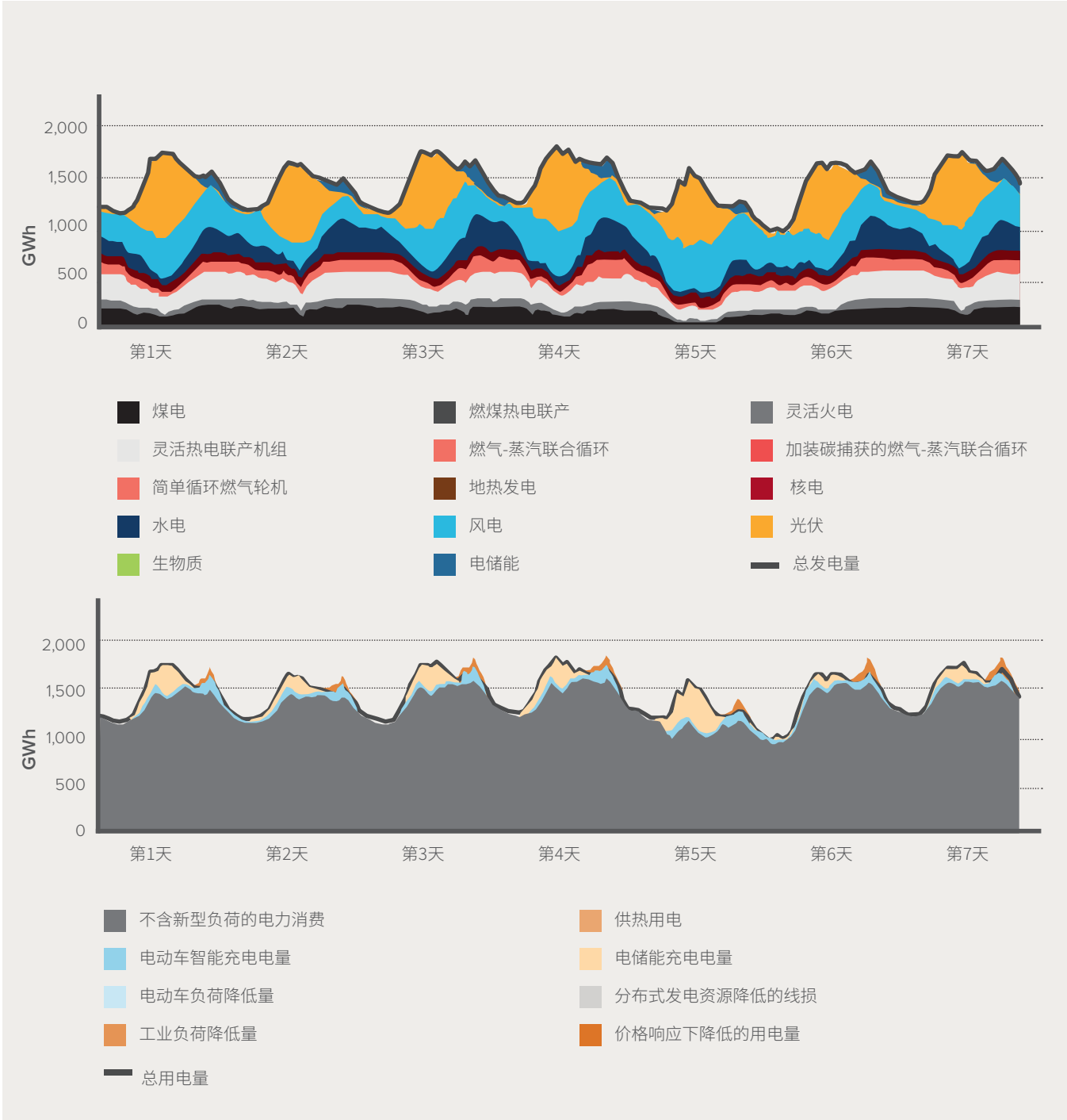
图 32 中国在2035年夏季的发电量与用电量预测曲线（既定政策情景） 40
